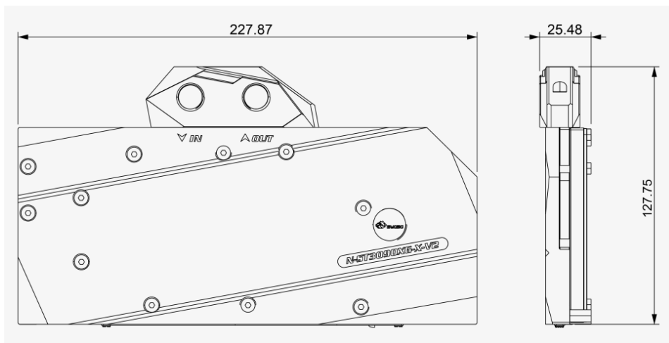
N-ST3090XG-X-V2 (1 pc)
