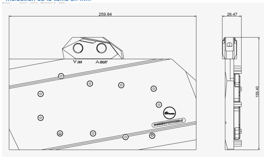
N-MS3070TRIO-X (1 pc)
