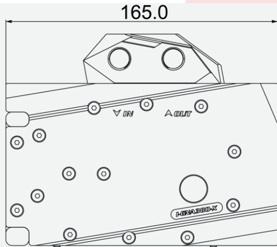
Waterblock (1 Stk.)
