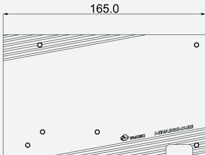
Backplate (1 Stk.)
